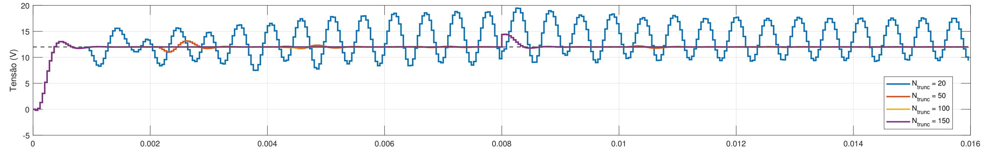
DMC — Variação de N_{\text{truncamento}}
